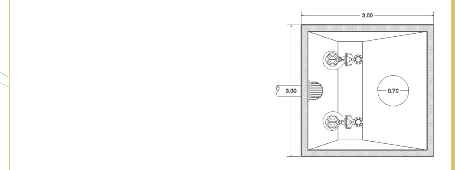
Pianta 1:50
