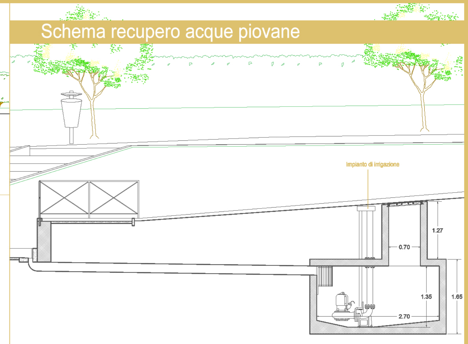
Sezione 1:50
